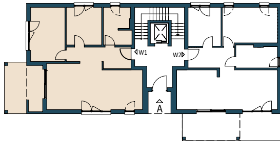
Erdgeschoss
